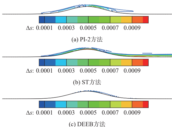
图 16 不同方法模拟得到的熵增云图
