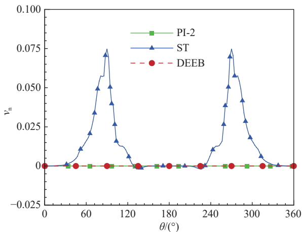
图 21 椭圆表面法向速度曲线
