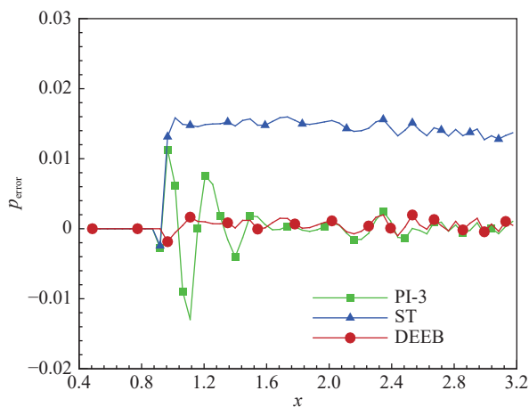
图 27 壁面压力误差曲线 Fig. 27 Relative error of the wall pressure
