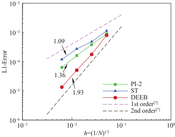
图 6 不同方法的熵增误差 L1 范数对比
