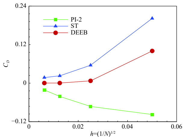
图 7 亚声速圆柱绕流阻力系数
