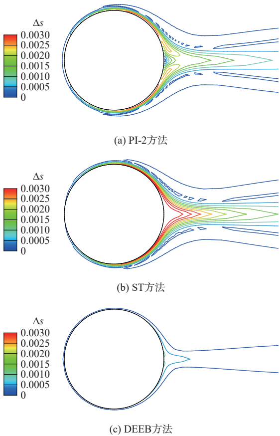
图 5 不同方法计算得到的熵增等值线图
