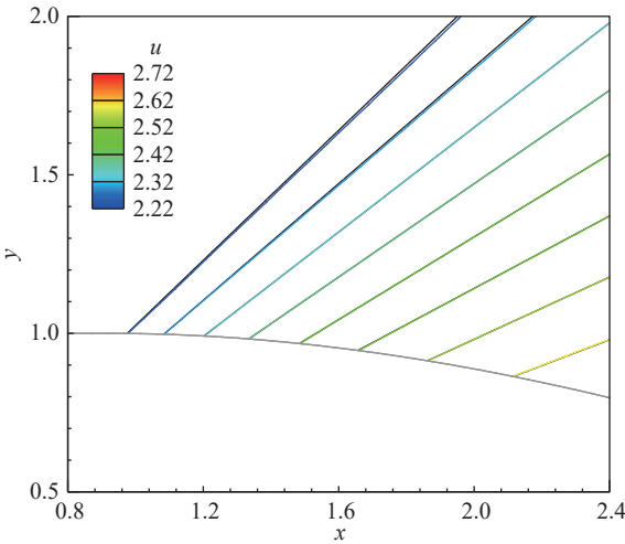
图 23 不同方法计算得到的速度 u 等值线图 Fig. 23 u contours obtained by different methods
