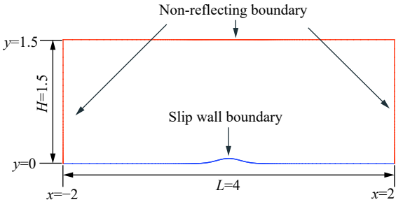
图 12 二维平滑凸起通道内亚声速流动计算边界
