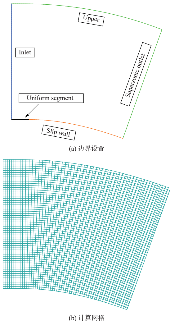
图 22 计算网格和边界条件设置
