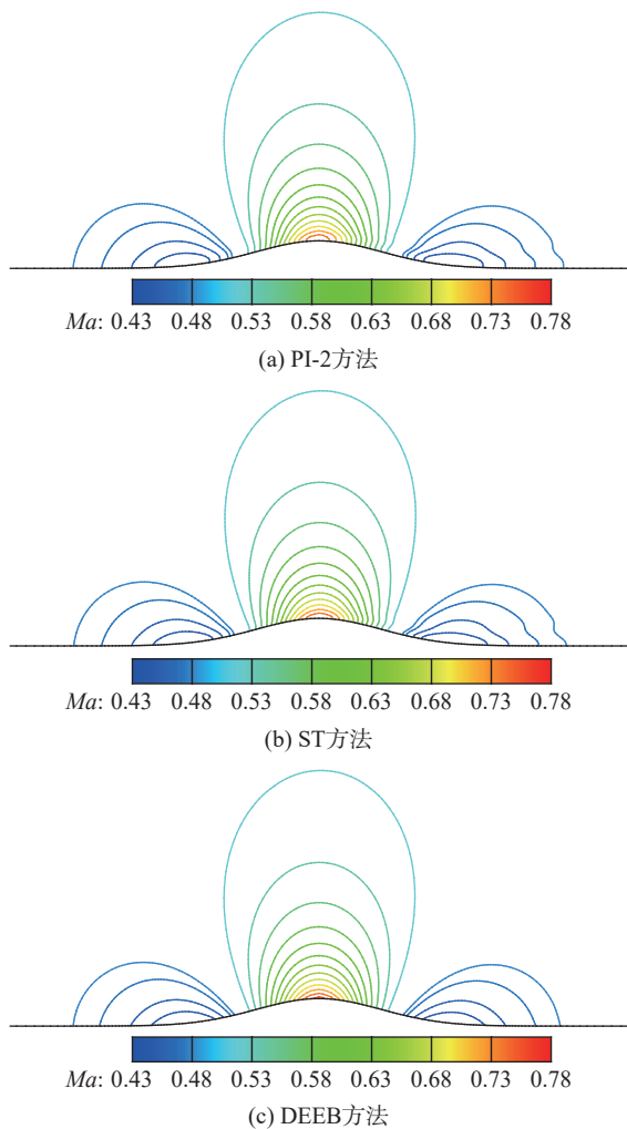
图 15 不同方法模拟得到的马赫数等值线图
