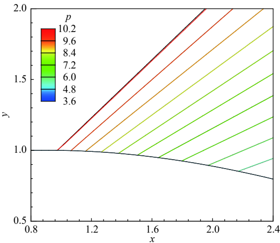
图 24 不同方法计算得到的压力等值线图 Fig. 24 Pressure contours obtained by different methods
