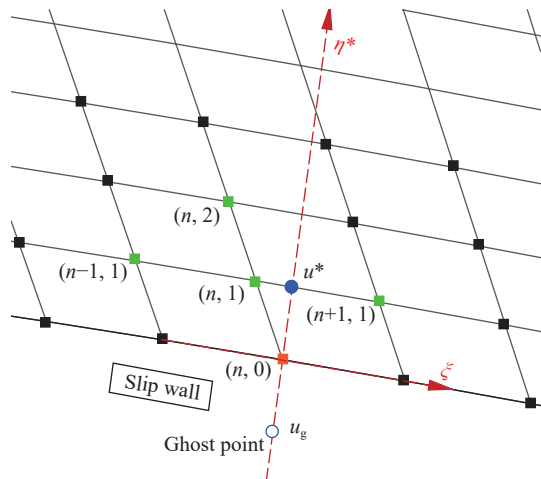
图3 非正交网格局部坐标系（一阶迎风格式）
