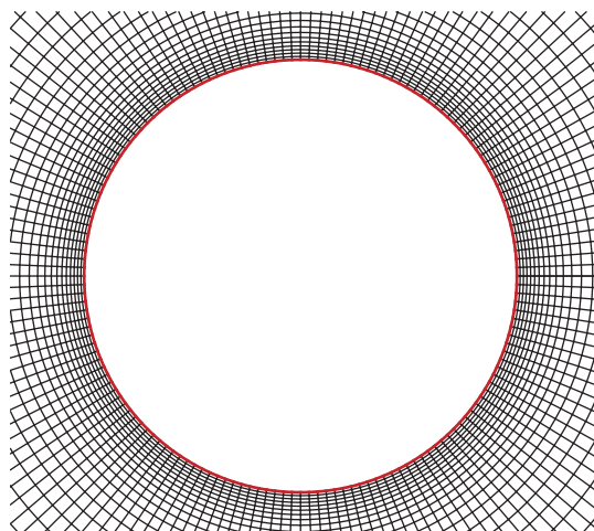
图 11 DEEB 算法激活区域 (Mesh3)
