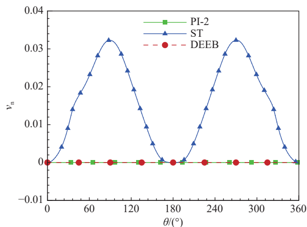
图 10 壁面法向速度分布曲线
