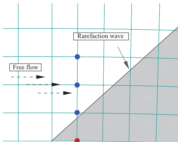
图 25 PI-3 方法外推插值误差分析 Fig. 25 Extrapolation error of PI-3 method
