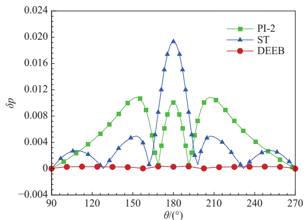
图 9 壁面上下游节点压力差分布曲线
