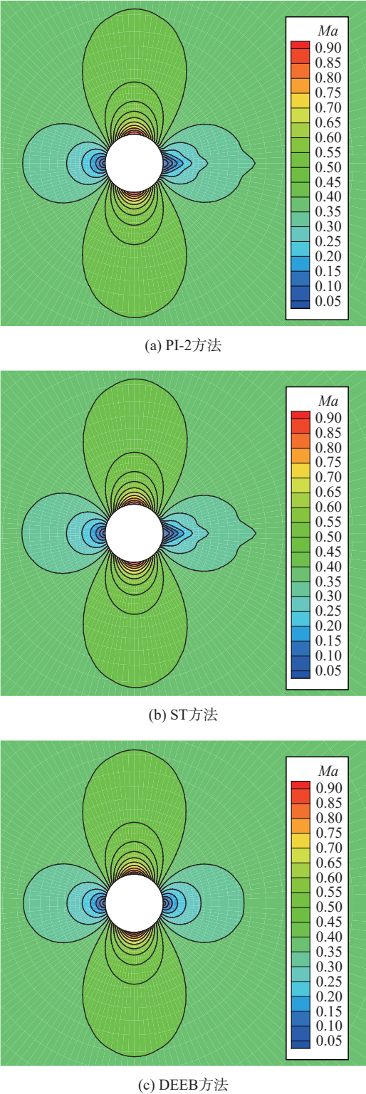
图 4 不同方法计算得到的马赫数等值线图
