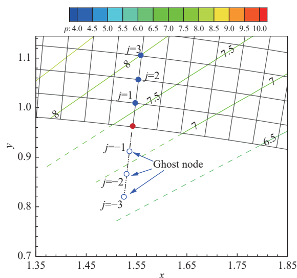
图 26 ST 方法虚拟节点构造误差分析 Fig. 26 Ghost node construction error of ST method
