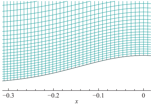
图 13 局部区域网格图
