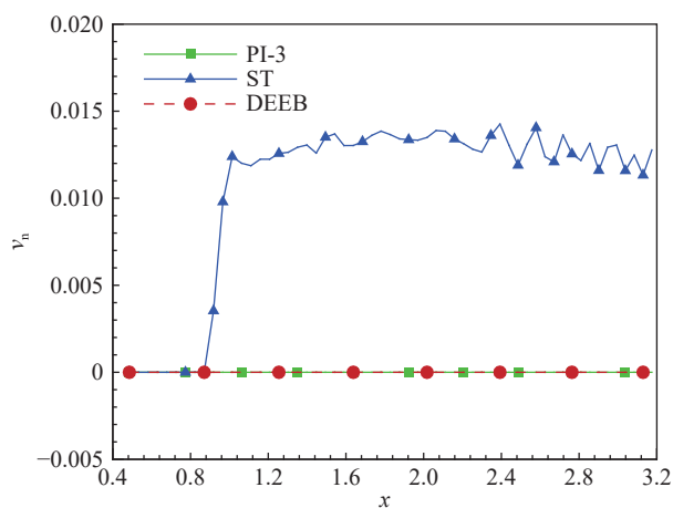
图 28 壁面法向速度曲线 Fig. 28 Surface wall-normal velocity
