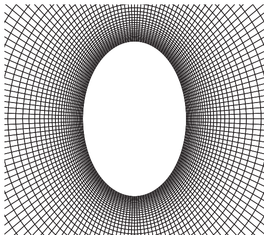
图 17 椭圆绕流局部网格图
