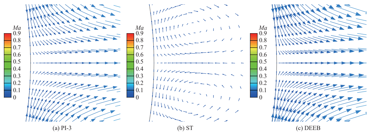
图 19 椭圆后缘绕流速度矢量图 Fig. 19 Velocity vectors at the trailing edge
