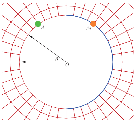
图 8 压力对称测点示意图
