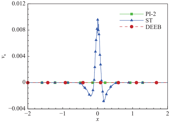
图 14 下壁面法向速度曲线
